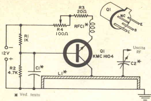
Fig. 1 - Nel trasmettitore viene usato un transistor speciale per microonde, il quale funziona come oscillatore di bassa potenza.
