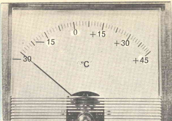
Fig. 2 - Usate le divisioni originali della scala dello strumento, ma cambiate la numerazione per indicare le graduazioni tra -30^{\circ}\text{C} e +45^{\circ}\text{C} ; sotto la nuova numerazione segnate la sigla della scala " ^{\circ}\text{C} ".
