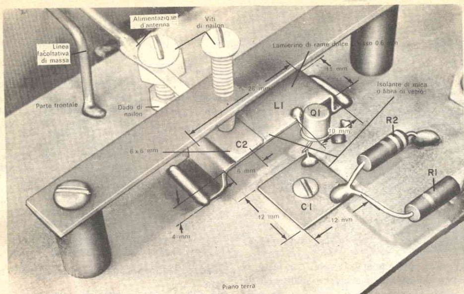
Fig. 3 - Costruzione meccanica del trasmettitore. Il condensatore per l'accoppiamento d'antenna (C2) ha il terminale stretto fissato tra la testa di una vite ed un dado, entrambi di nailon. Per costruire il ponte di supporto per la vite di accordo, potrete usare un pezzo di basetta per circuiti stampati, filettando il foro per C2 con una vite metallica.
