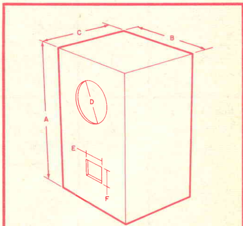
Fig. 3 - Mobile universale consigliato da T. W. Richardson per altoparlanti di cui non sono note le caratteristiche. Si accordi il mobile a 40 Hz e si usi legno compensato da 2 cm ben rinforzato con listelli, incollando ed avvitando insieme le parti con blocchetti agli angoli. Il volume dovrebbe essere di almeno 0,14 m 3 . I valori tipici per le dimensioni A, B e C saranno rispettivamente di 76 cm - 53 cm - 37 cm. Se non si dispone di strumenti di prova, si adotti un valore di 10 cm per E e 9 cm per F.
