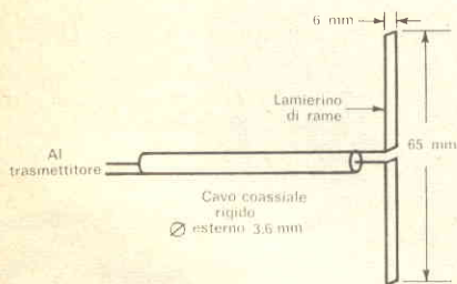
Fig. 9 - Per sperimentare vari tipi di antenna, può essere usato questo semplice dipolo. Altre antenne potranno essere a fascio, a tromba o paraboliche. Per installare questa antenna occorre staccare quella vecchia ed il piano terra.
