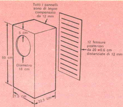
Fig. 4 - Questo mobile compatto (da 28 dm 3 ) per altoparlanti da 20 cm ha tutti i pannelli interni imbottiti con materiale fonosorbente spesso 25 mm. Il pannello posteriore è imbottito con stoffa morbida. Le fessure possono essere fatte tagliando strisce di legno compensato spesso 12 mm nella giusta larghezza e montandole su una cornice alla distanza di 12 mm l'una dall'altra. Si possono anche praticare serie di fori da 12 mm di diametro per ottenere la stessa area della fessura da 20x0,6 cm.
