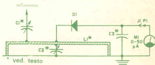
Fig. 6 - Nel ricevitore, a causa delle altissime frequenze in gioco, viene usato un diodo speciale per microonde. Le polarità del diodo sono indifferenti, purché lo strumento che misura il livello del segnale indichi nel giusto senso.
