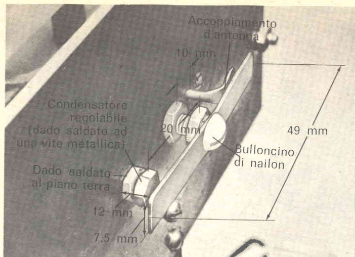
Fig. 5 - L'accoppiamento d'antenna viene effettuato (da C2 del trasmettitore) praticando una zona piana ad un'estremità di un tondino di rame dolce. Per eseguire questa operazione, ruotate l'antenna di 90°. Dopo il montaggio, l'accoppiamento di antenna deve essere vicino a quest'ultima, senza però che tocchi l'antenna stessa.
