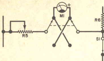
Fig. 4 - Aggiungendo un commutatore per l'inversione della polarità dello strumento, il termometro si può usare anche per temperature inferiori a -30^{\circ}\text{C} .
