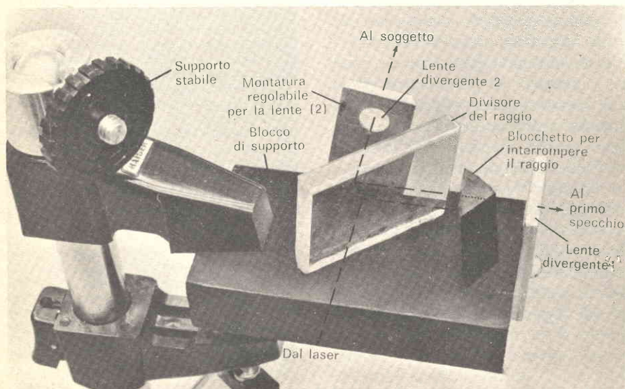
Fig. 2 - Particolari del complesso divisore del raggio. Il blocchetto opaco è disposto in modo da interrompere uno dei raggi provenienti dal divisore. Le lenti divergenti si devono orientare opportunamente nell'area del raggio laser.
