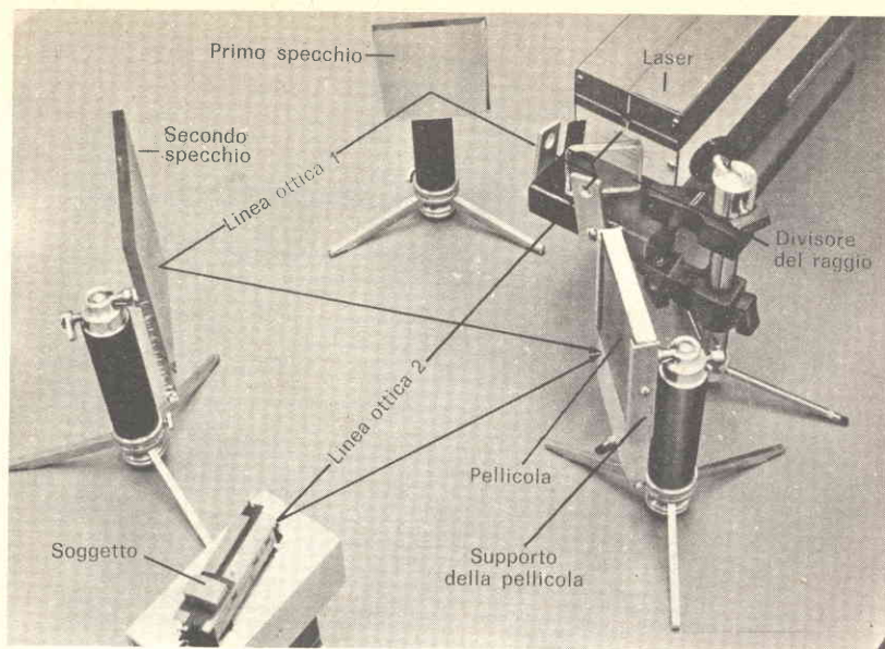
Fig. 1 - Complesso ottico usato per fare un ologramma. I treppiedi sono del tipo normale usato in fotografia. Si tenga presente che la cosa più importante è la stabilità assoluta sia del raggio laser sia delle altre parti ottiche.
